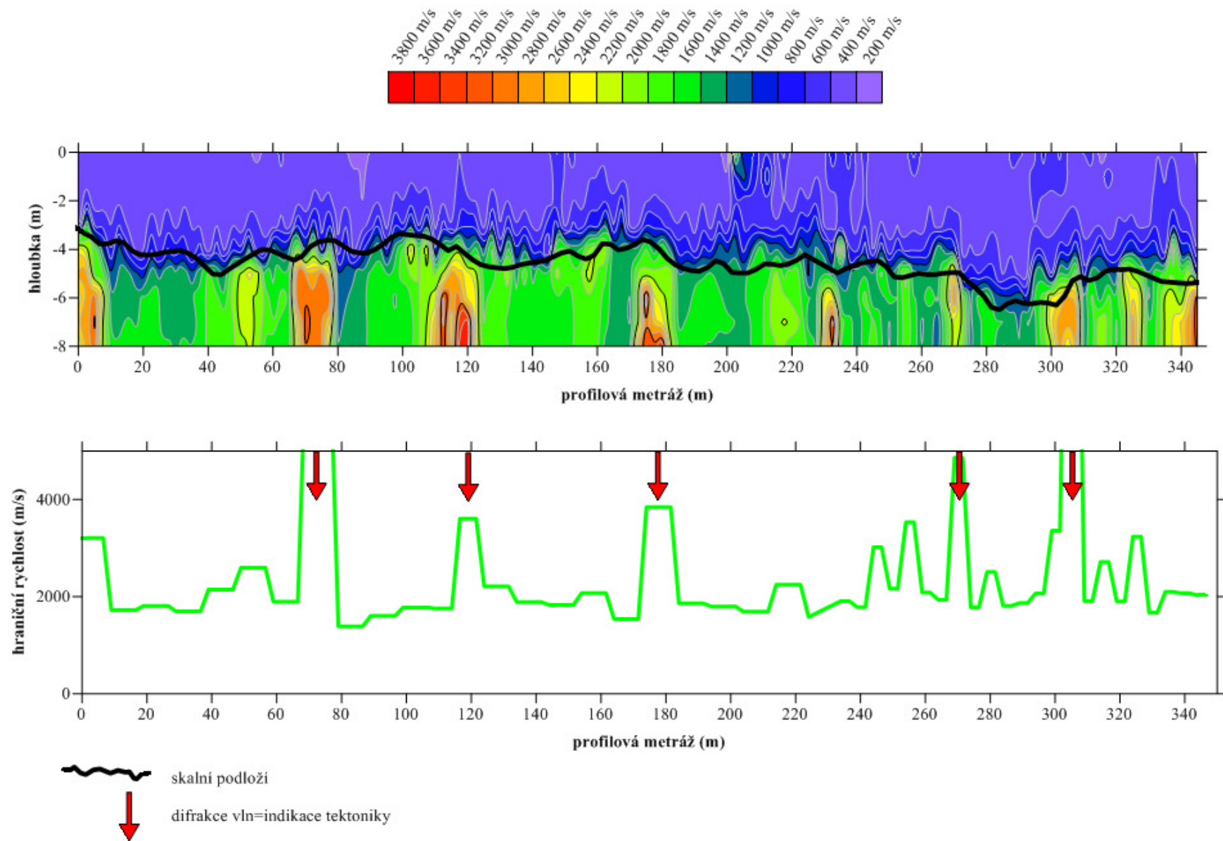
Obr. 2: Seismický řez S1 a graf hraničních rychlostí s indikacemi tektoniky
